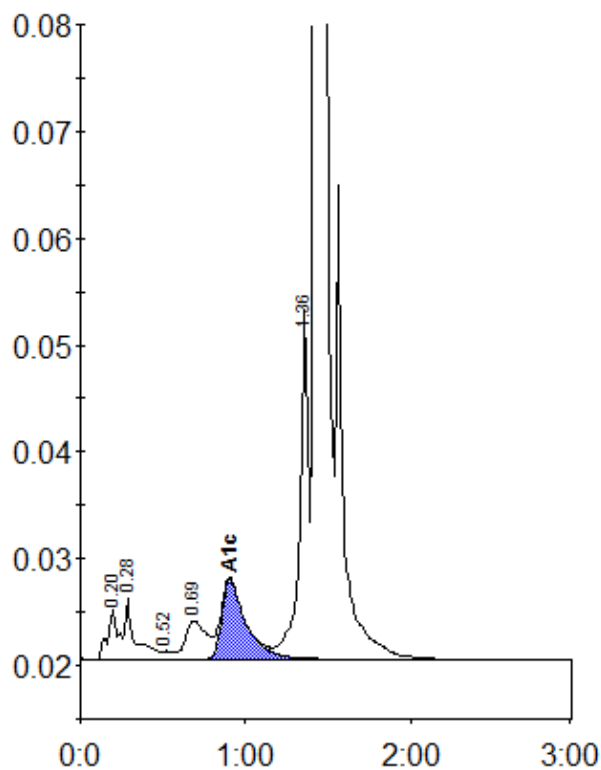
Peak table - ID: 10409788
